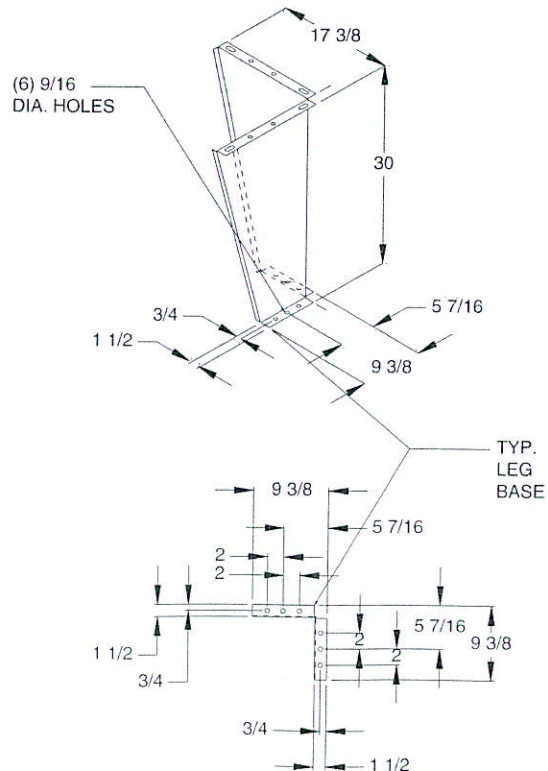
Optional 30 inch leg
